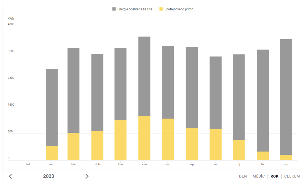
Graf: spotřeba energie ČOV – šedě energie dodaná ze sítě, žlutě energie vyrobená FVE
